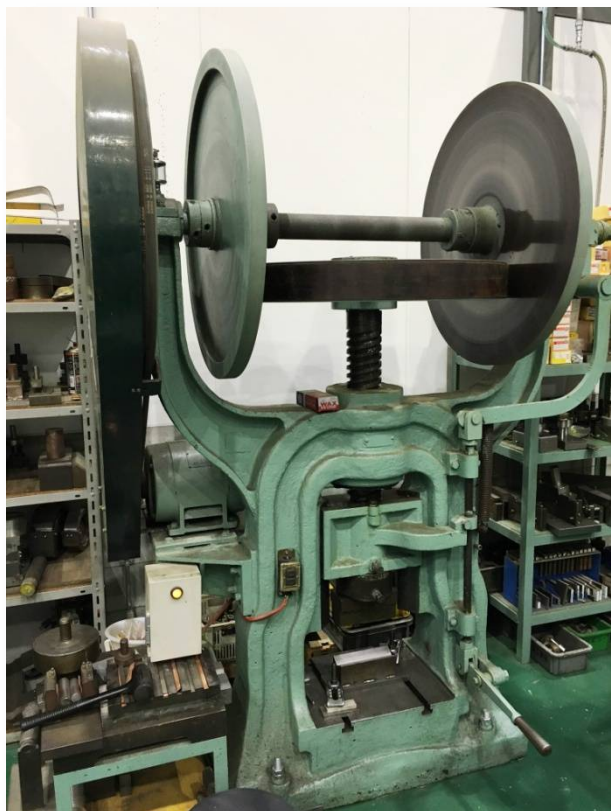
フレキシオンプレス (森鉄工所 150t)
